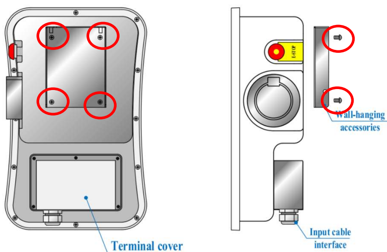
Figure 8 Fixation des accessoires d'accrochage mural
