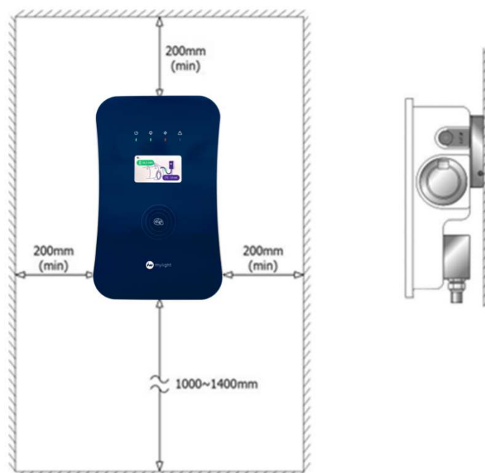
Figure 6 Espace minimum requis pour le montage mural
