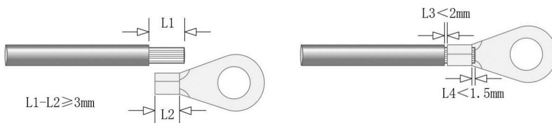
Figure 9 : Dénuder les câbles et presser les terminaux
