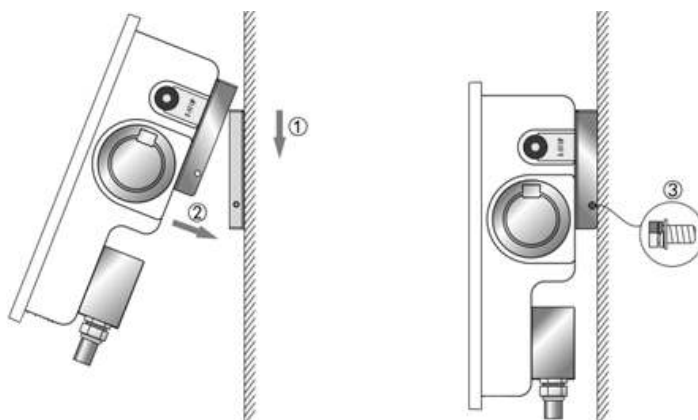
Figure 11 Fixation de la borne au mur
