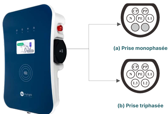
Figure 1 Schéma de la prise de type 2 sur les produits
